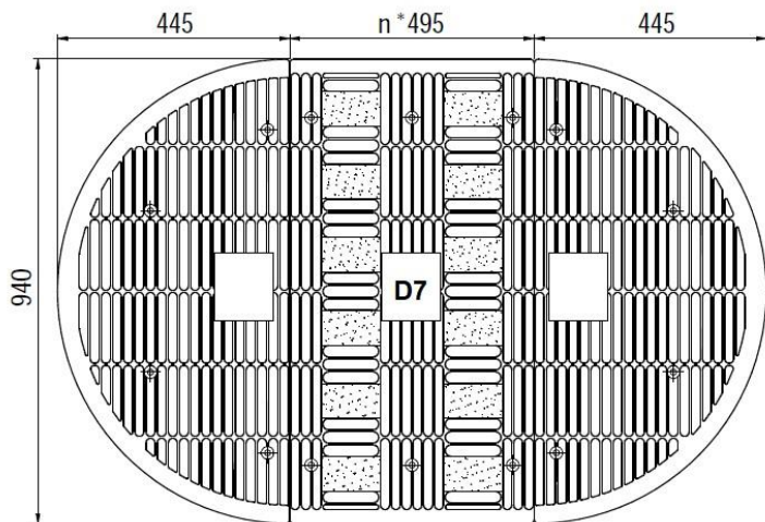
Liniowy próg zwalniający D7
