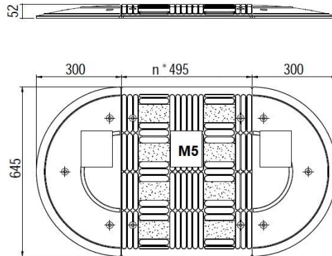
Liniowy próg zwalniający M5
