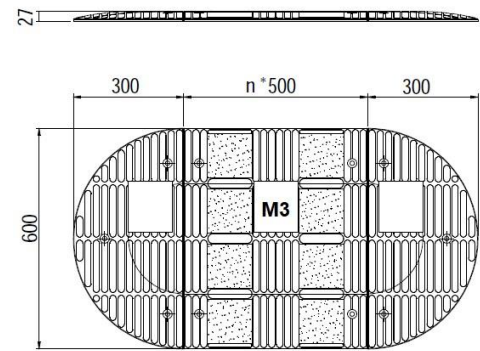
Liniowy próg zwalniający M3
