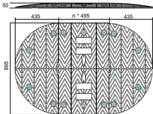
Liniowy próg zwalniający D5 Eco/ Premium
