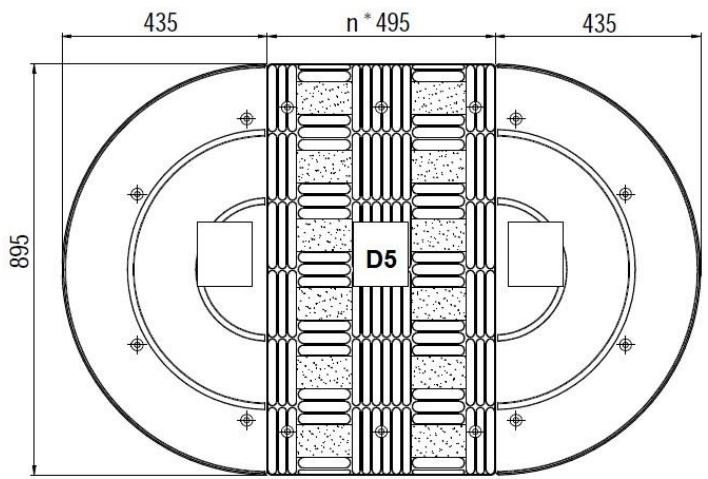
Liniowy próg zwalniający D5
